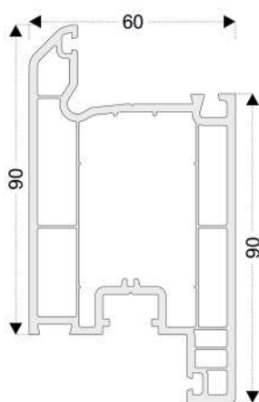
PRO04 Inward Door Profile
